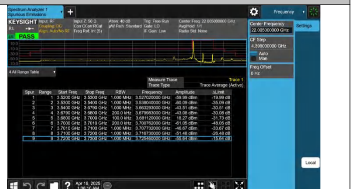
Band48-20MHz-QPSK-56640-1RB#0-PASS
