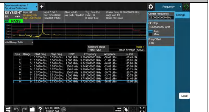
Band48-20MHz-QPSK-55340-1RB#99-PASS
