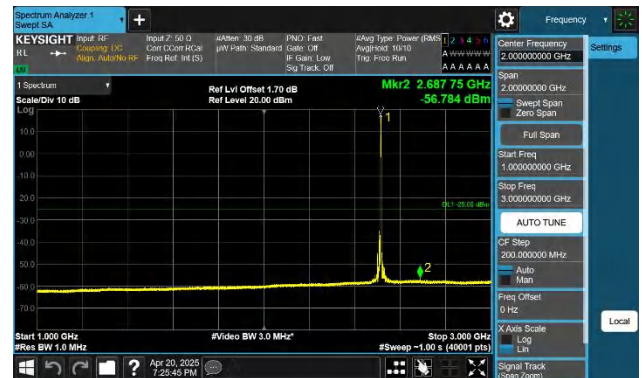
41-41-20MHz-10MHz-QPSK-QPSK-39750-39894-1RB#99-ORB#0 -1000~3000MHz-PASS
