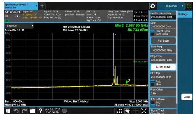
41-41-20MHz-15MHz-QPSK-QPSK-39750-39921-1RB#0-0RB#0 1000~3000MHz-PASS
