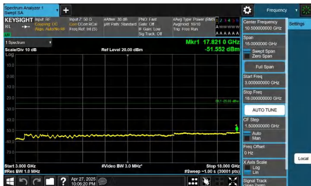
41-41-20MHz-20MHz-QPSK-QPSK-40521-40719-1RB#0-0RB#0 -3000~18000MHz-PASS
