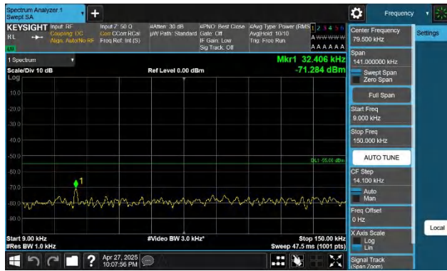
41-41-20MHz-20MHz-QPSK-QPSK-41292-41490-1RB#0-0RB#0 -0.009~0.15MHz-PASS
