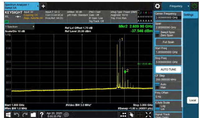
41-41-20MHz-20MHz-QPSK-QPSK-39750-39948-1RB#0-1RB#99 -1000~3000MHz-PASS
