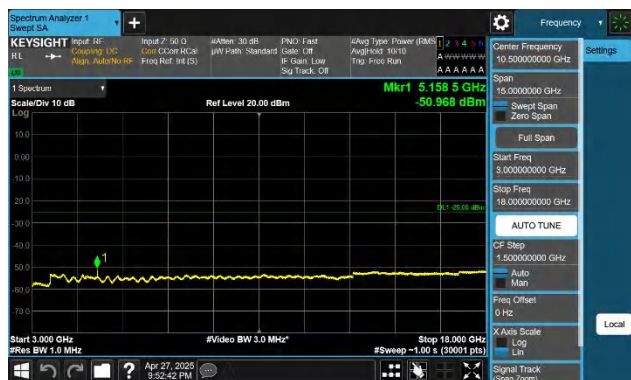
41-41-20MHz-10MHz-QPSK-QPSK-40571-40715-1RB#0-0RB#0 -3000~18000MHz-PASS
