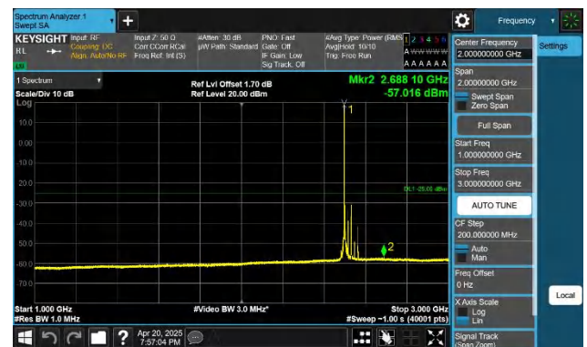
41-41-20MHz-20MHz-QPSK-QPSK-39750-39948-1RB#0-0RB#0 1000~3000MHz-PASS
