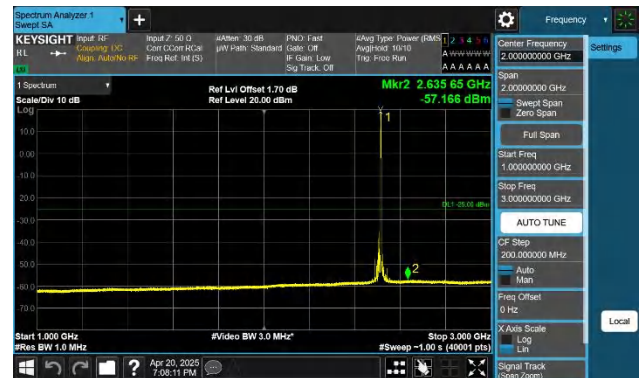
41-41-20MHz-5MHz-QPSK-QPSK-39750-39867-1RB#99-0RB#0 1000~3000MHz-PASS
