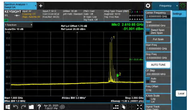
41-41-20MHz-5MHz-QPSK-QPSK-39750-39867-1RB#0-1RB#24- 1000~3000MHz-PASS
