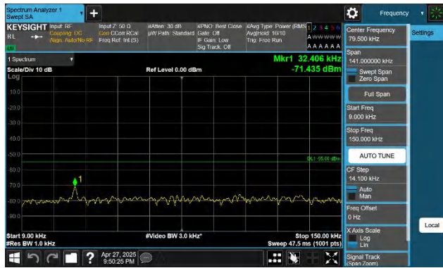
41-41-20MHz-10MHz-QPSK-QPSK-39750-39894-1RB#0-0RB#0 -0.009~0.15MHz-PASS
