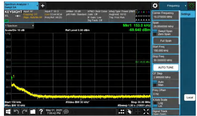
41-41-20MHz-5MHz-QPSK-QPSK-39750-39867-1RB#0-0RB#0-0. 15~30MHz-PASS
