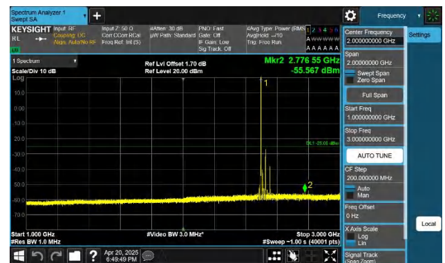
41-41-15MHz-20MHz-QPSK-QPSK-39728-39899-1RB#0-0RB#0 1000~3000MHz-PASS
