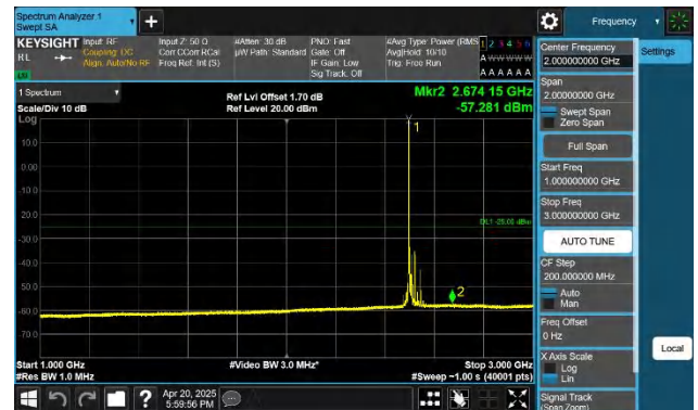
41-41-10MHz-20MHz-QPSK-QPSK-39705-39849-1RB#0-0RB#0 1000~3000MHz-PASS
