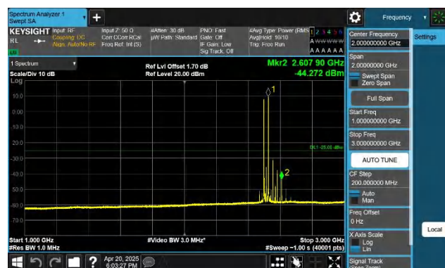
41-41-10MHz-20MHz-QPSK-QPSK-39705-39849-1RB#0-1RB#99 -1000~3000MHz-PASS
