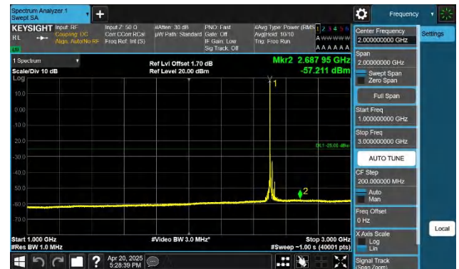
41-41-5MHz-20MHz-QPSK-QPSK-39683-39800-1RB#24-0RB#0 1000~3000MHz-PASS
