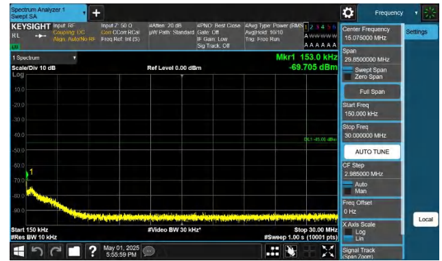
41-41-5MHz-20MHz-QPSK-QPSK-39683-39800-1RB#24-0RB#0 0.15~30MHz-PASS
