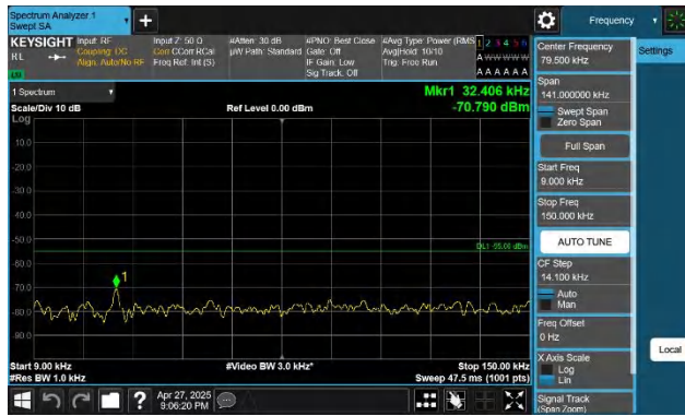
41-41-5MHz-20MHz-QPSK-QPSK-40528-40645-1RB#0-0RB#0- 0.009~0.15MHz-PASS
