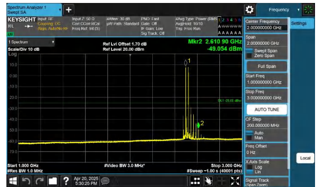
41-41-5MHz-20MHz-QPSK-QPSK-39683-39800-1RB#0-1RB#99- 1000~3000MHz-PASS
