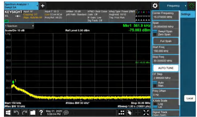
41-41-5MHz-20MHz-QPSK-QPSK-40528-40645-1RB#24-0RB#0 0.15~30MHz-PASS
