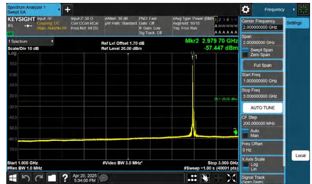
41-41-5MHz-20MHz-QPSK-QPSK-40528-40645-1RB#24-0RB#0 1000~3000MHz-PASS
