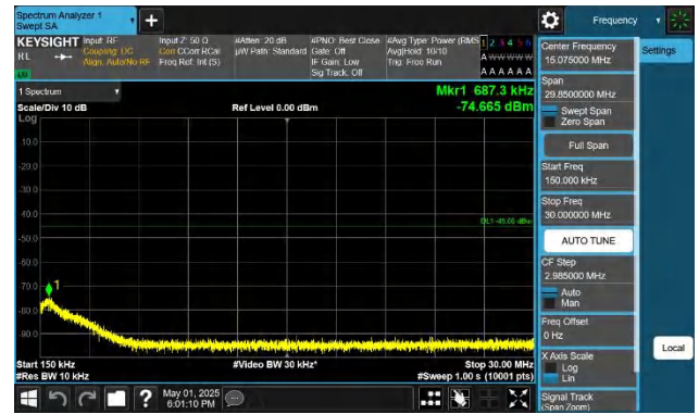
41-41-5MHz-20MHz-QPSK-QPSK-41373-41490-1RB#0-1RB#99- 0.15~30MHz-PASS
