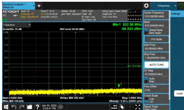
7-7-20MHz-15MHz-QPSK-QPSK-21026-21197-1RB#0-0RB#0-30 ~1000MHz-PASS
