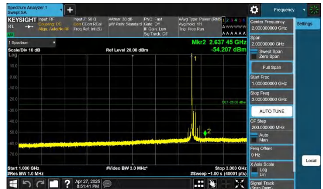
7-7-20MHz-15MHz-QPSK-QPSK-21026-21197-1RB#0-0RB#0-10 00~3000MHz-PASS
