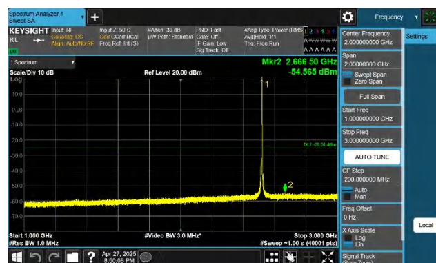
7-7-20MHz-15MHz-QPSK-QPSK-20850-21021-1RB#99-0RB#0-1 000~3000MHz-PASS
