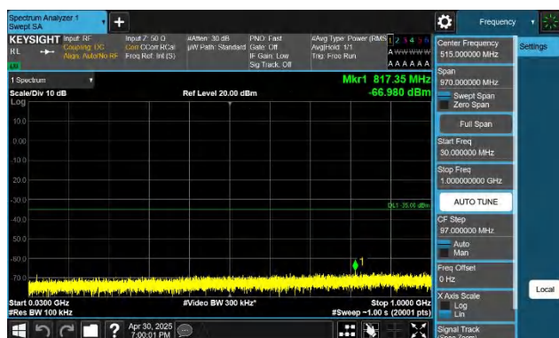
7-7-20MHz-15MHz-QPSK-QPSK-21026-21197-1RB#99-ORB#0-3 0~1000MHz-PASS
