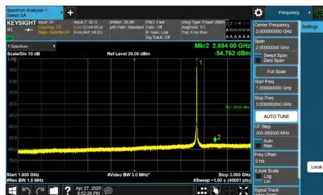
7-7-20MHz-15MHz-QPSK-QPSK-21026-21197-1RB#99-ORB#0-1 000~3000MHz-PASS
