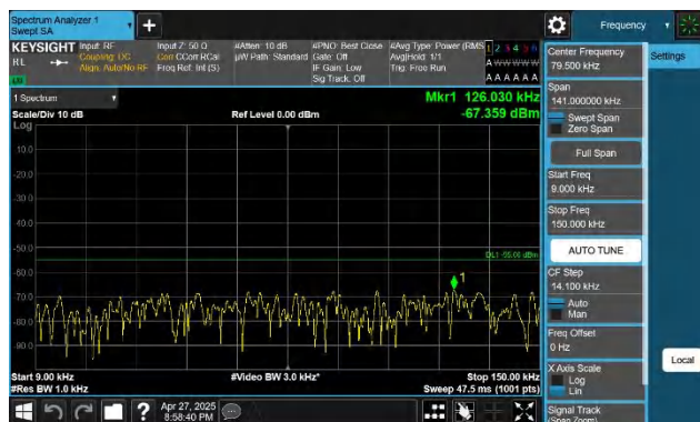
7-7-20MHz-20MHz-QPSK-QPSK-21001-21199-1RB#0-0RB#0-0. 009~0.15MHz-PASS
