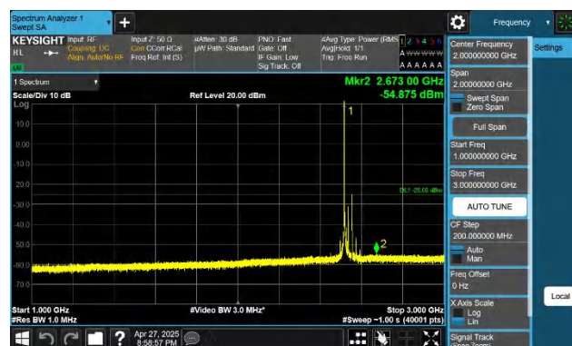
7-7-20MHz-20MHz-QPSK-QPSK-21001-21199-1RB#0-0RB#0-10 00~3000MHz-PASS
