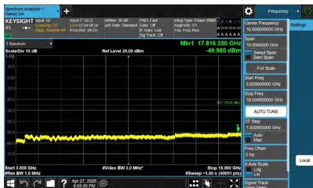
7-7-20MHz-15MHz-QPSK-QPSK-21201-21372-1RB#0-1RB#74- 3000~18000MHz-PASS
