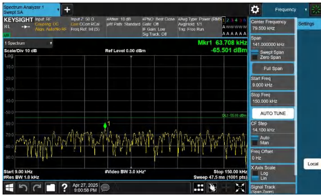
7-7-20MHz-20MHz-QPSK-QPSK-21152-21350-1RB#0-0RB#0-0. 009~0.15MHz-PASS
