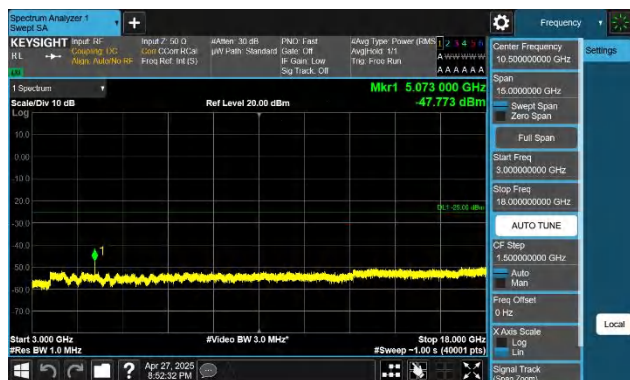
7-7-20MHz-15MHz-QPSK-QPSK-21026-21197-1RB#99-ORB#0-3 000~18000MHz-PASS
