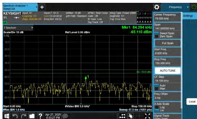
7-7-15MHz-20MHz-QPSK-QPSK-20828-20999-1RB#0-0RB#0-0. 009~0.15MHz-PASS
