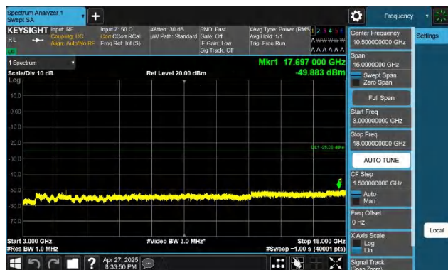
7-7-15MHz-20MHz-QPSK-QPSK-20828-20999-1RB#0-0RB#0-3 000~18000MHz-PASS
