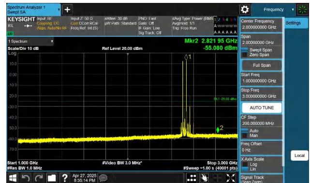
7-7-15MHz-20MHz-QPSK-QPSK-20828-20999-1RB#0-1RB#99-1 000~3000MHz-PASS
