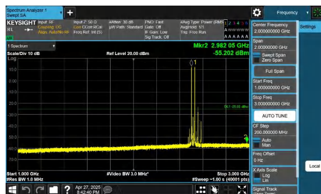
7-7-20MHz-10MHz-QPSK-QPSK-20850-20994-1RB#0-1RB#49-1 000~3000MHz-PASS
