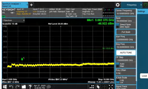
7-7-20MHz-10MHz-QPSK-QPSK-21251-21395-1RB#0-0RB#0-3 000~18000MHz-PASS
