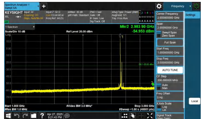
7-7-15MHz-10MHz-QPSK-QPSK-21051-21171-1RB#0-1RB#49-1 000~3000MHz-PASS
