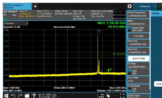
7-7-10MHz-20MHz-QPSK-QPSK-21006-21150-1RB#0-1RB#99-1 000~3000MHz-PASS
