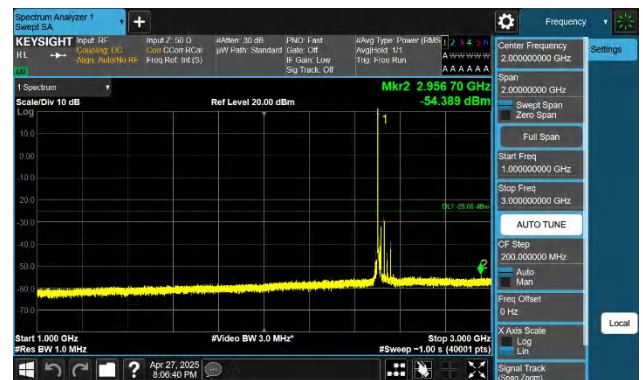
7-7-10MHz-20MHz-QPSK-QPSK-20805-20949-1RB#0-ORB#0-10 00~3000MHz-PASS
