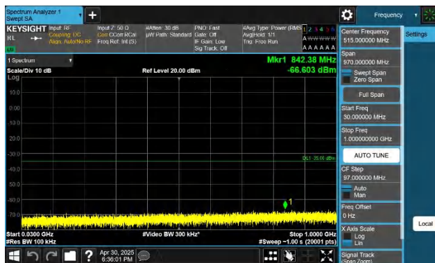
7-7-10MHz-20MHz-QPSK-QPSK-20805-20949-1RB#0-ORB#0-3 0~1000MHz-PASS
