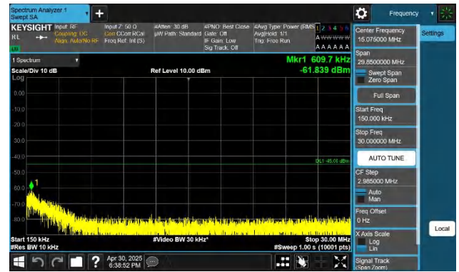
7-7-10MHz-20MHz-QPSK-QPSK-21206-21350-1RB#0-1RB#99-0. 15~30MHz-PASS
