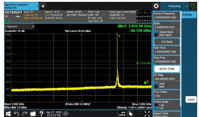
7-7-10MHz-20MHz-QPSK-QPSK-20805-20949-1RB#49-ORB#0-1.000~3000MHz-PASS
