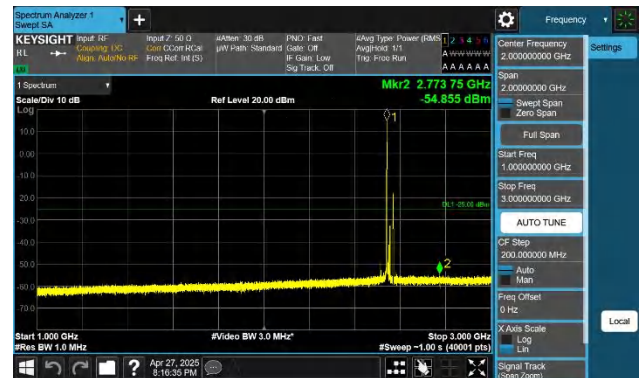
7-7-10MHz-20MHz-QPSK-QPSK-21206-21350-1RB#0-1RB#99-1 000~3000MHz-PASS
