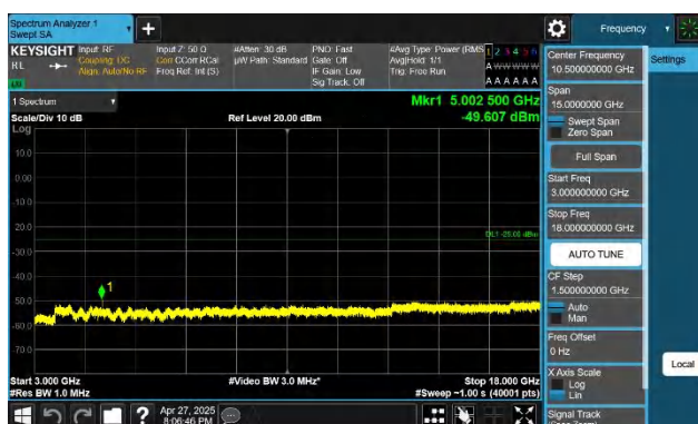
7-7-10MHz-20MHz-QPSK-QPSK-20805-20949-1RB#0-ORB#0-3 000~18000MHz-PASS
