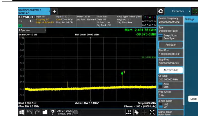
5-5-10MHz-10MHz-QPSK-QPSK-20476-20575-1RB#0-0RB#0-10 00~3000MHz-PASS
