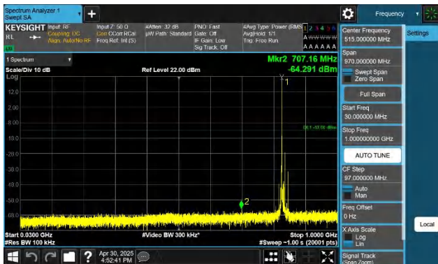
5-5-10MHz-10MHz-QPSK-QPSK-20501-20600-1RB#0-0RB#0-30 ~1000MHz-PASS
