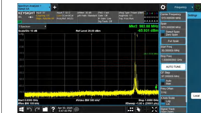
5-5-10MHz-5MHz-QPSK-QPSK-20500-20572-1RB#0-ORB#0-30~ 1000MHz-PASS
