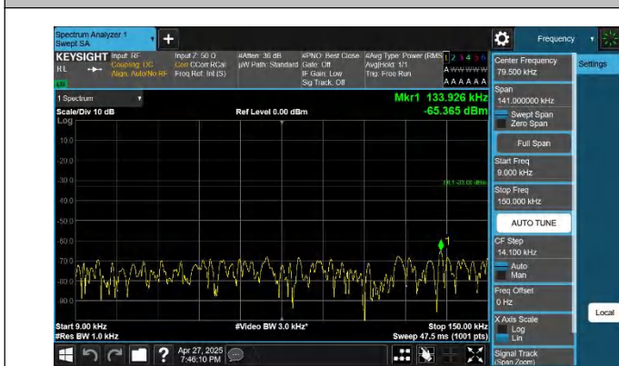
5-5-5MHz-10MHz-QPSK-QPSK-20428-20500-1RB#24-0RB#0-0. 009~0.15MHz-PASS
