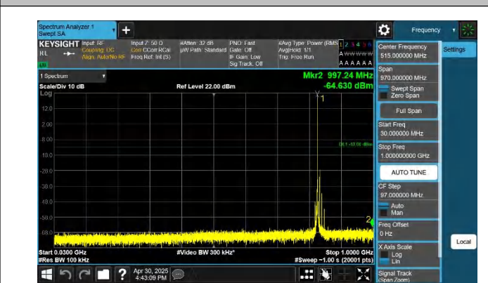
5-5-5MHz-10MHz-QPSK-QPSK-20478-20550-1RB#0-ORB#0-30~ 1000MHz-PASS
