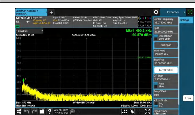
5-5-5MHz-10MHz-QPSK-QPSK-20428-20500-1RB#24-0RB#0-0. 15~30MHz-PASS
