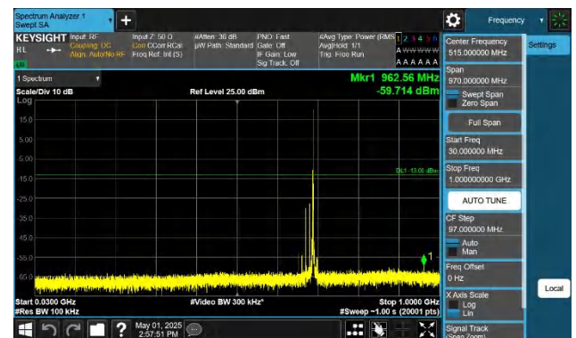
Band71-20MHz-QPSK-133372-1RB#99-30~1000-PASS
