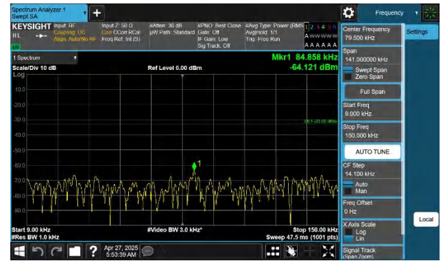
Band71-20MHz-QPSK-133372-1RB#99-0.009~0.15-PASS
