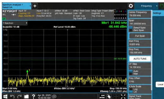
Band66-20MHz-QPSK-132572-1RB#0-0.009~0.15-PASS
