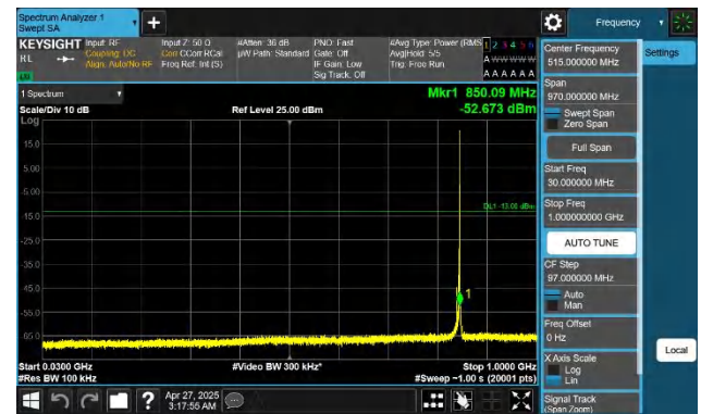
Band26(824-849)-3MHz-QPSK-27025-1RB#14-30~1000-PASS
