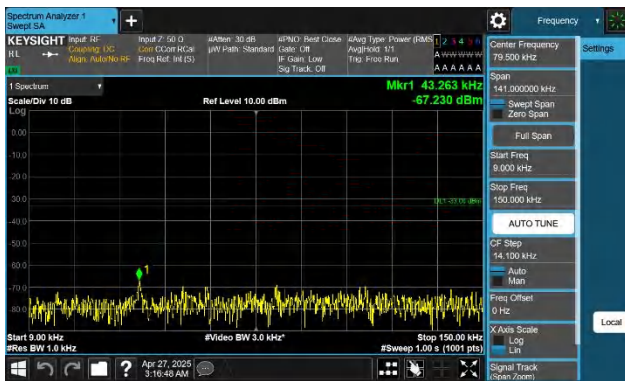
Band26(824-849)-3MHz-QPSK-27025-1RB#0-0.009~0.15-PASS
