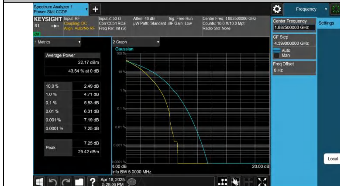
Band25-5MHz-QPSK-26365-25RB#0-PASS
