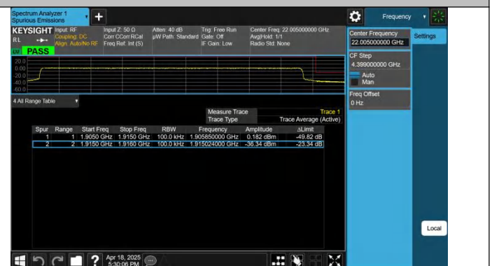
Band25-10MHz-QPSK-26640-50RB#0-PASS
