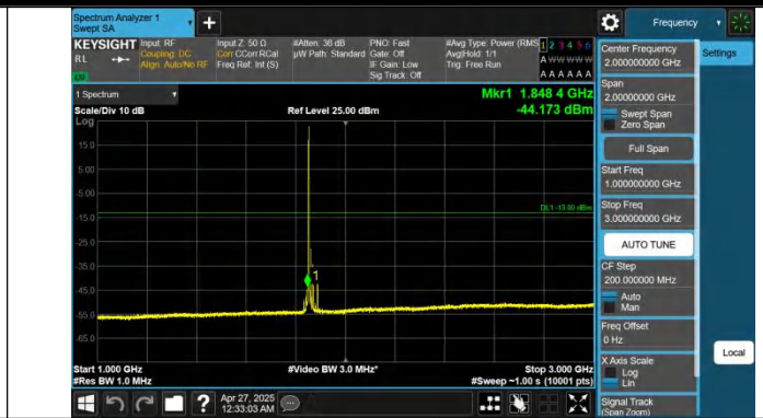
Band2-20MHz-QPSK-18700-1RB#0-1000~3000-PASS
