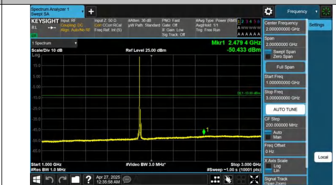
Band2-20MHz-QPSK-19100-1RB#0-1000~3000-PASS
