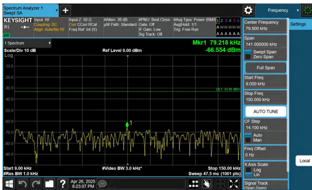
Band71-20MHz-QPSK-133372-1RB#0-0.009~0.15-PASS
