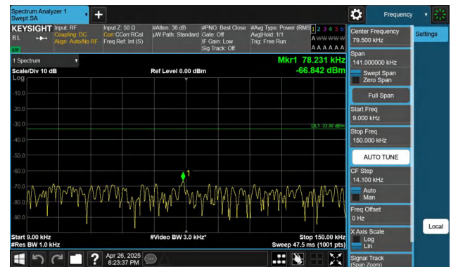
Band71-20MHz-QPSK-133372-1RB#99-0.009~0.15-PASS
