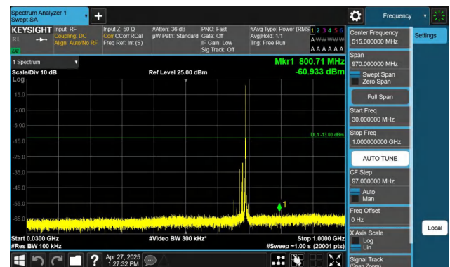
Band71-20MHz-QPSK-133372-1RB#99-30~1000-PASS
