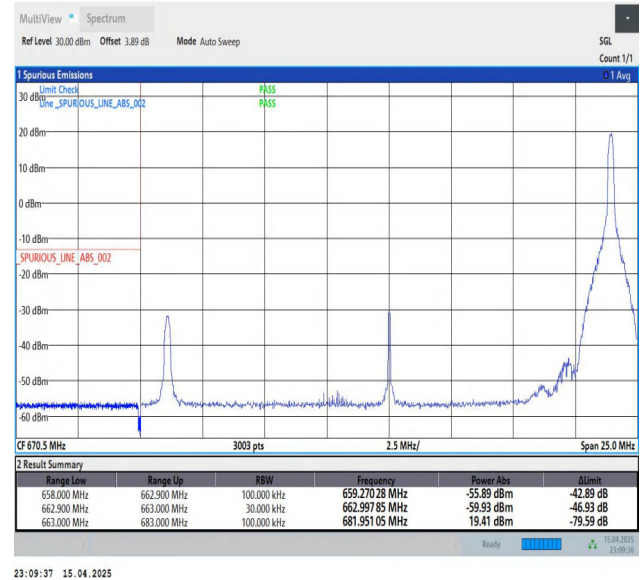
Band71-20MHz-QPSK-133222-1RB#99-PASS
