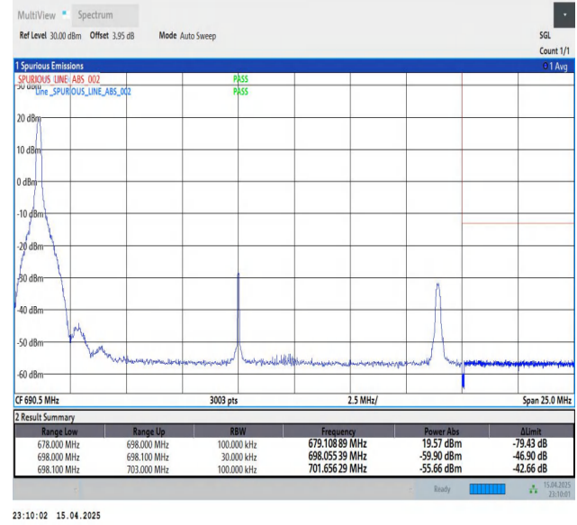
Band71-20MHz-QPSK-133372-1RB#0-PASS
