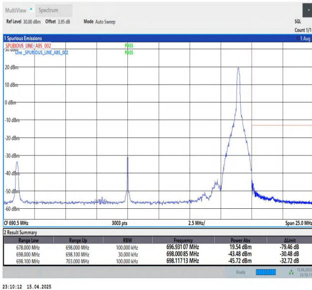
Band71-20MHz-QPSK-133372-1RB#99-PASS
