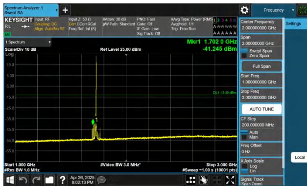
Band66-20MHz-QPSK-132072-1RB#99-1000~3000-PASS
