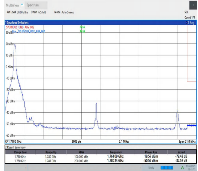
Band66-20MHz-QPSK-132572-1RB#0-PASS
