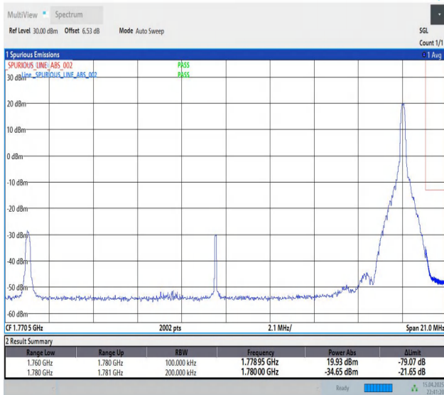
Band66-20MHz-QPSK-132572-1RB#99-PASS
