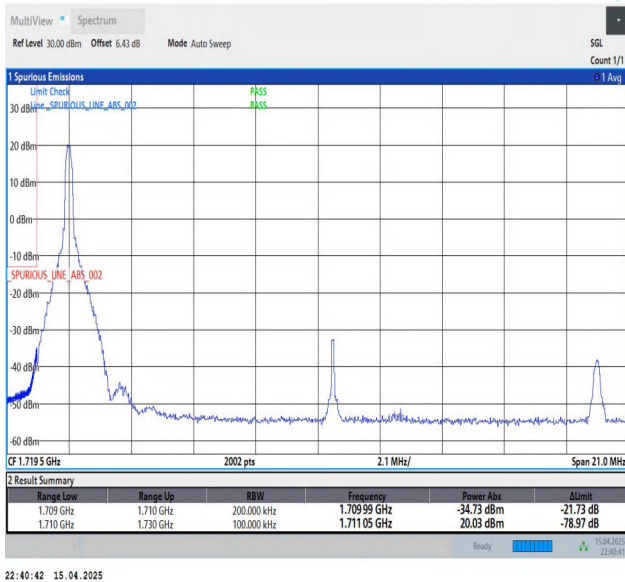
Band66-20MHz-QPSK-132072-1RB#0-PASS
