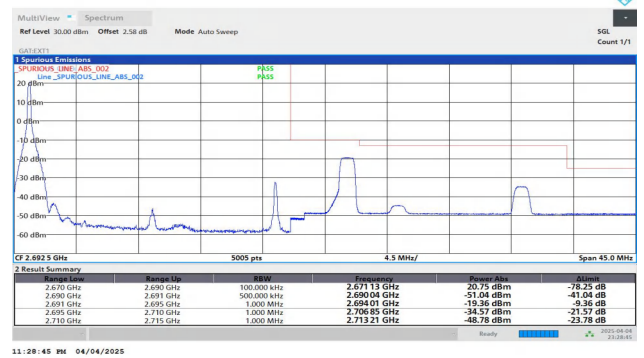
Band41-20MHz-QPSK-41490-1RB#0-PASS
