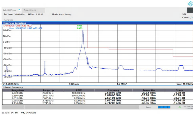
Band41-20MHz-QPSK-41490-1RB#99-PASS
