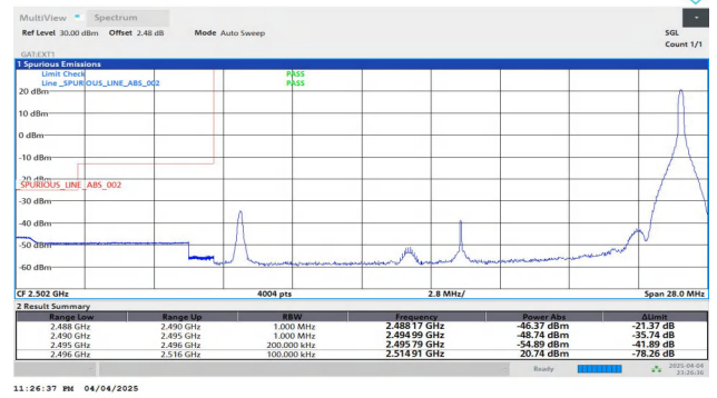
Band41-20MHz-QPSK-39750-1RB#99-PASS
