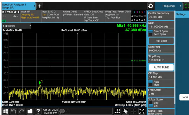
Band26(824-849)-10MHz-QPSK-26990-1RB#0-0.009~0.15-PASS
