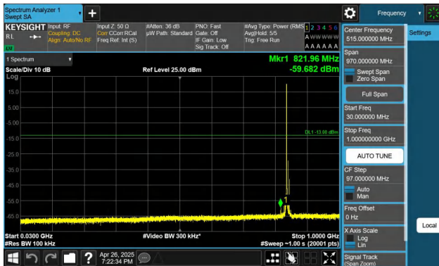
Band26(824-849)-10MHz-QPSK-26990-1RB#0-30~1000-PASS
