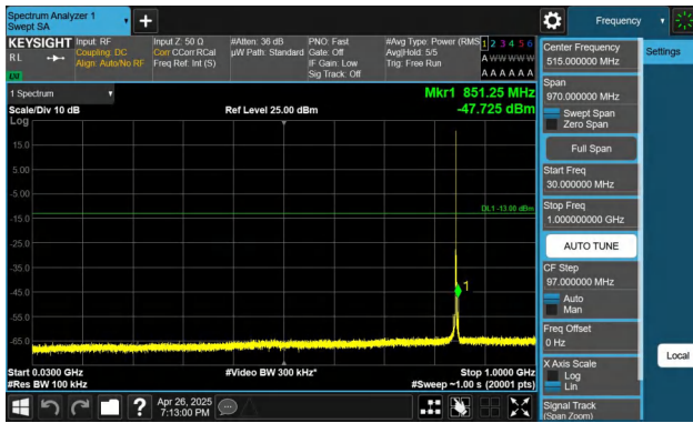
Band26(824-849)-3MHz-QPSK-27025-1RB#0-30~1000-PASS
