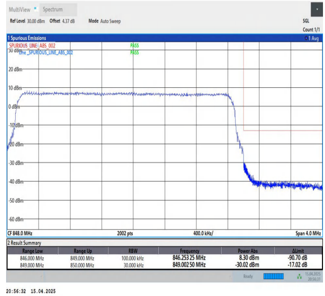
Band26(824-849)-3MHz-QPSK-27025-15RB#0-PASS
