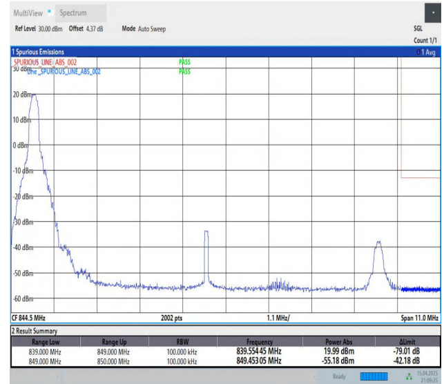
Band26(824-849)-10MHz-QPSK-26990-1RB#0-PASS
