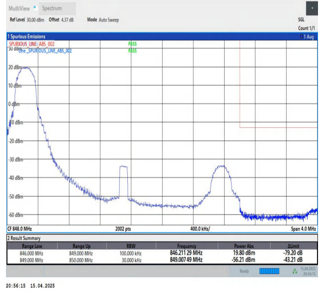
Band26(824-849)-3MHz-QPSK-27025-1RB#0-PASS
