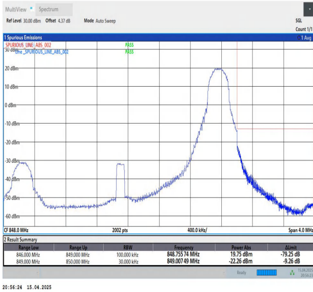
Band26(824-849)-3MHz-QPSK-27025-1RB#14-PASS
