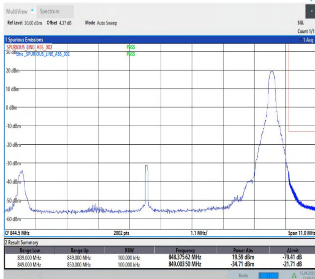
Band26(824-849)-10MHz-QPSK-26990-1RB#49-PASS
