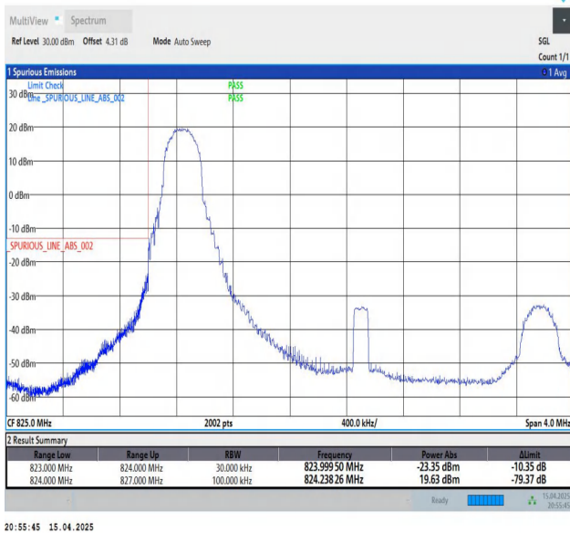
Band26(824-849)-3MHz-QPSK-26805-1RB#0-PASS
