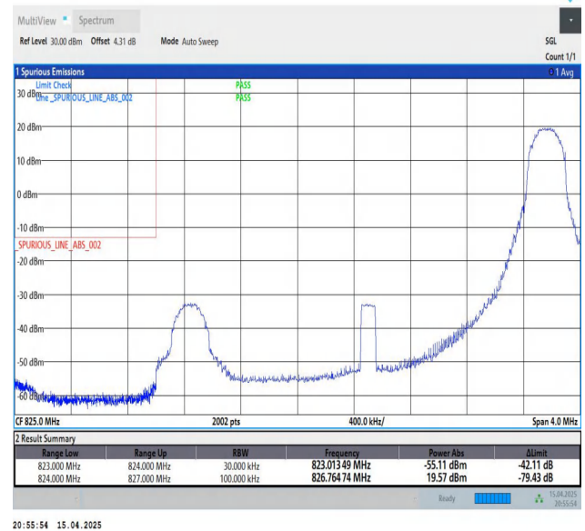
Band26(824-849)-3MHz-QPSK-26805-1RB#14-PASS
