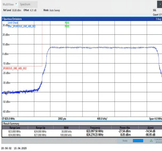
Band26(824-849)-3MHz-QPSK-26805-15RB#0-PASS
