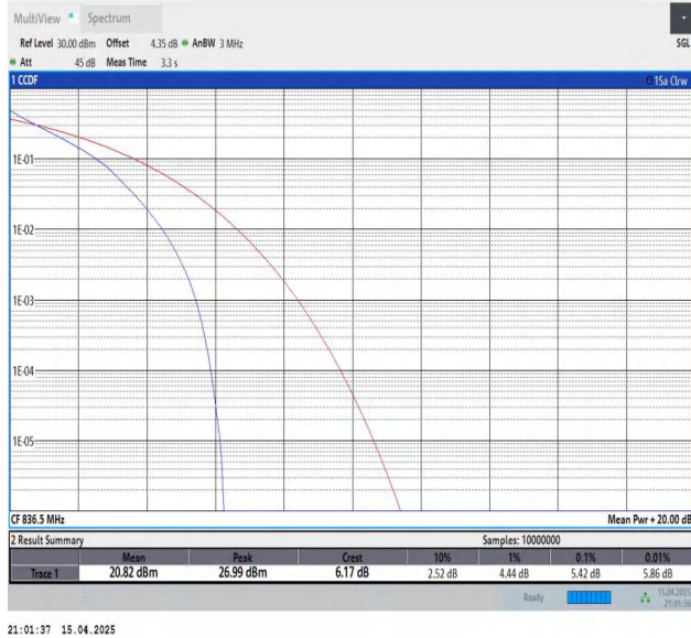
Band26(824-849)-3MHz-QPSK-26915-15RB#0-PASS
