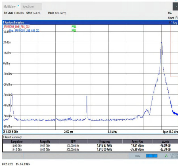
Band25-20MHz-QPSK-26590-1RB#99-PASS
