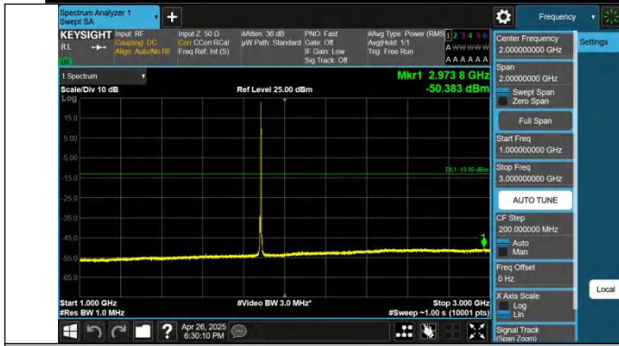
Band25-3MHz-QPSK-26365-1RB#14-1000~3000-PASS
