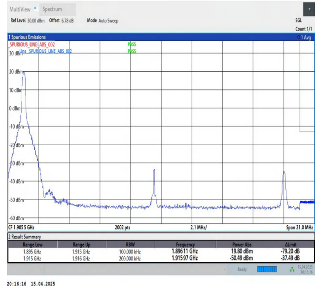
Band25-20MHz-QPSK-26590-1RB#0-PASS
