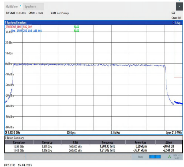
Band25-20MHz-QPSK-26590-100RB#0-PASS
