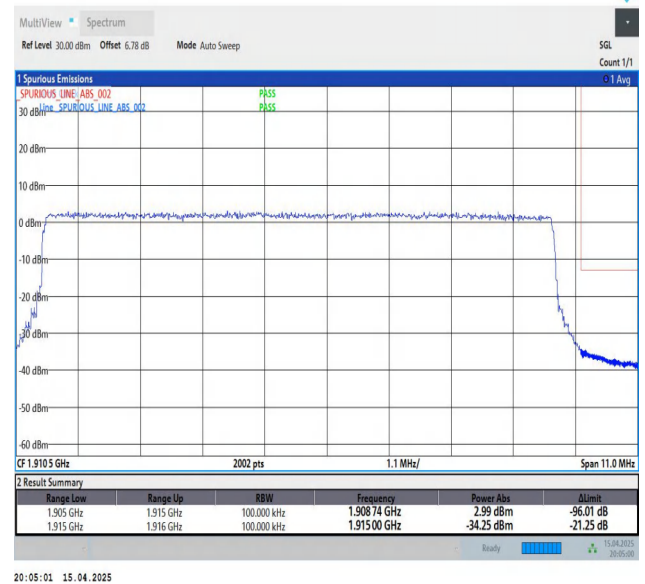
Band25-10MHz-QPSK-26640-50RB#0-PASS
