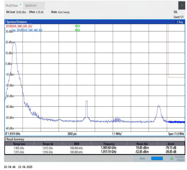
Band25-10MHz-QPSK-26640-1RB#0-PASS
