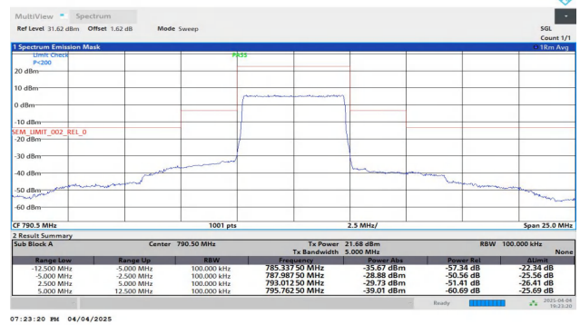
NTNV-Band14-5MHz-QPSK-23305-25RB#0--5.00--2.50-PASS
