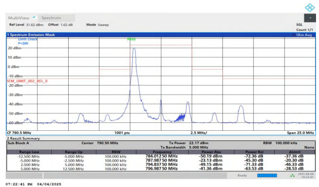
NTNV-Band14-5MHz-QPSK-23305-1RB#0--5.00--2.50-PASS
