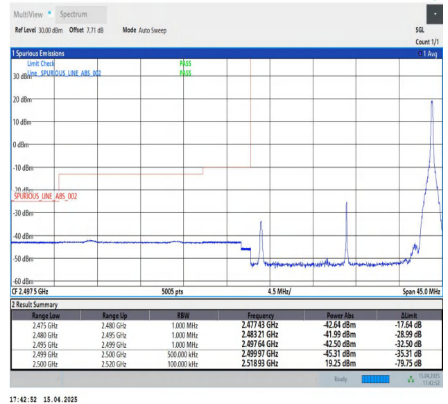
Band7-20MHz-QPSK-20850-1RB#99-PASS
