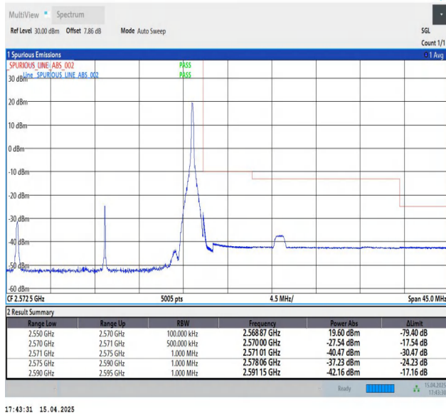
Band7-20MHz-QPSK-21350-1RB#99-PASS
