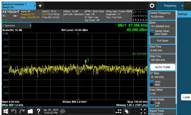
Band4-20MHz-QPSK-20175-1RB#0-0.009~0.15-PASS
