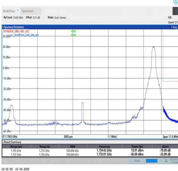
Band4-10MHz-QPSK-20350-1RB#49-PASS
