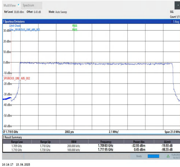
Band4-20MHz-QPSK-20050-100RB#0-PASS
