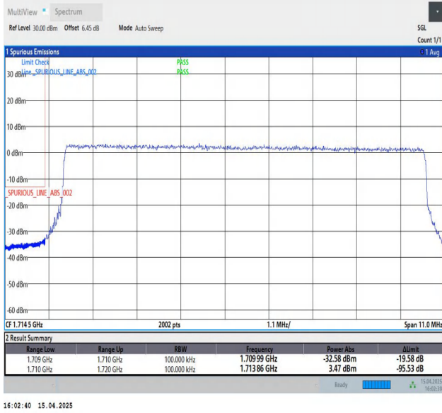
Band4-10MHz-QPSK-20000-50RB#0-PASS
