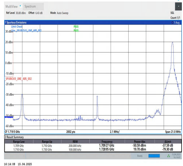
Band4-20MHz-QPSK-20050-1RB#99-PASS
