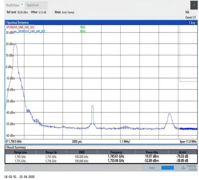
Band4-10MHz-QPSK-20350-1RB#0-PASS
