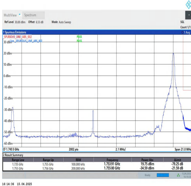
Band4-20MHz-QPSK-20300-1RB#99-PASS
