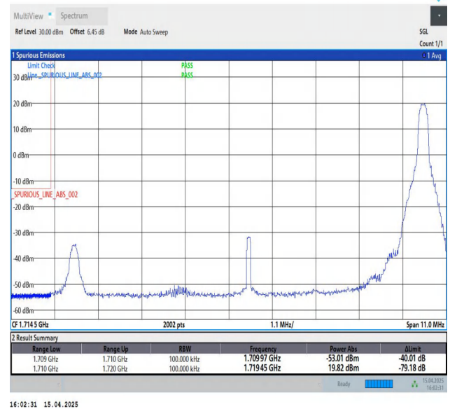
Band4-10MHz-QPSK-20000-1RB#49-PASS
