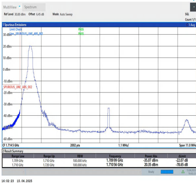
Band4-10MHz-QPSK-20000-1RB#0-PASS
