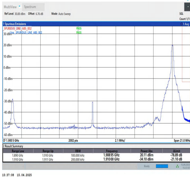
Band2-20MHz-QPSK-19100-1RB#99-PASS
