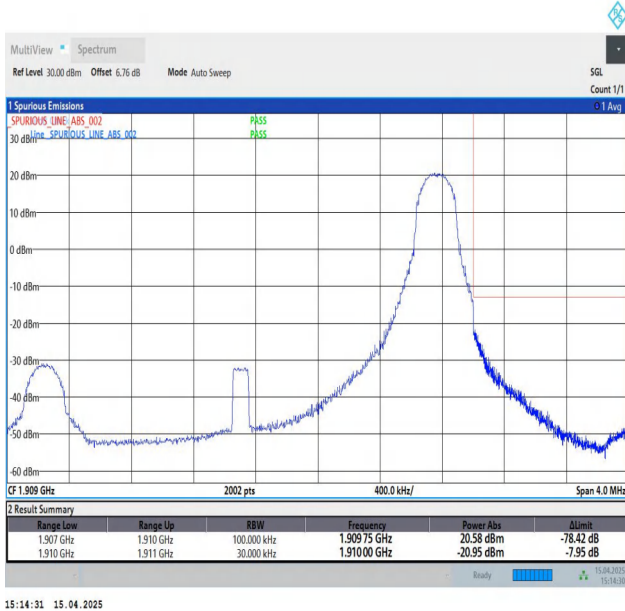
Band2-3MHz-QPSK-19185-1RB#14-PASS
