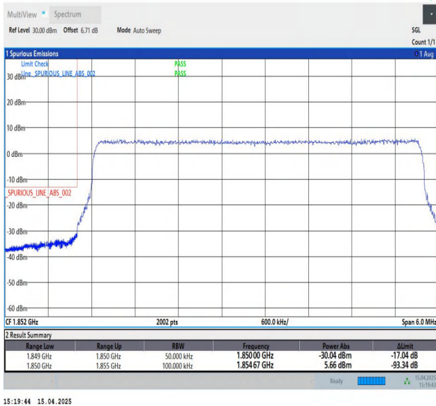
Band2-5MHz-QPSK-18625-25RB#0-PASS
