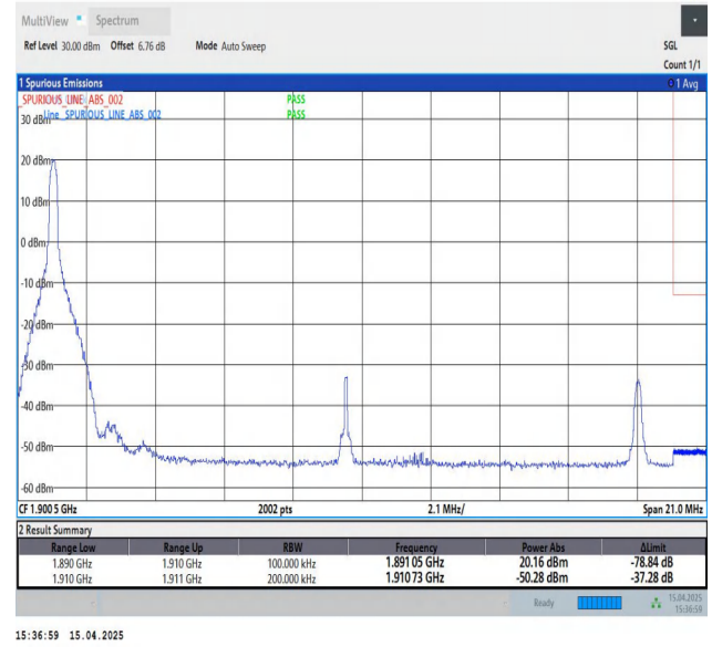
Band2-20MHz-QPSK-19100-1RB#0-PASS
