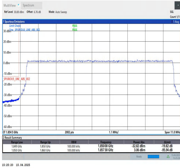
Band2-10MHz-QPSK-18650-50RB#0-PASS
