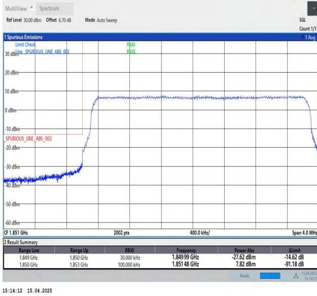
Band2-3MHz-QPSK-18615-15RB#0-PASS
