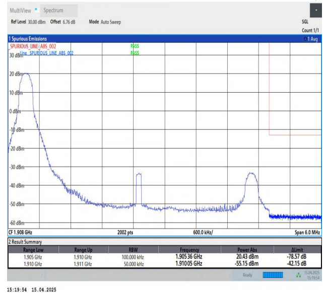
Band2-5MHz-QPSK-19175-1RB#0-PASS
