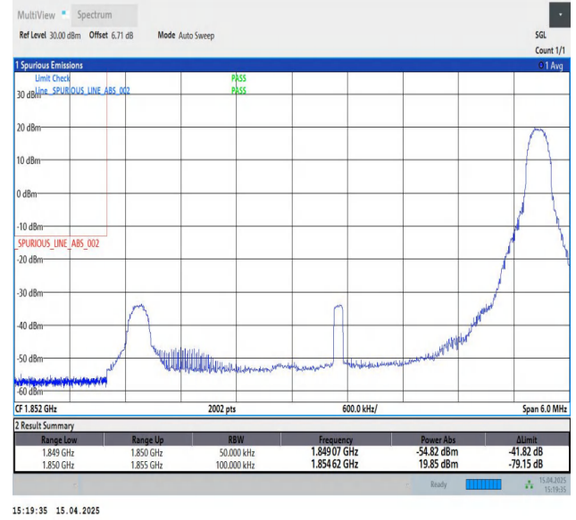
Band2-5MHz-QPSK-18625-1RB#24-PASS
