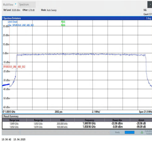
Band2-20MHz-QPSK-18700-100RB#0-PASS
