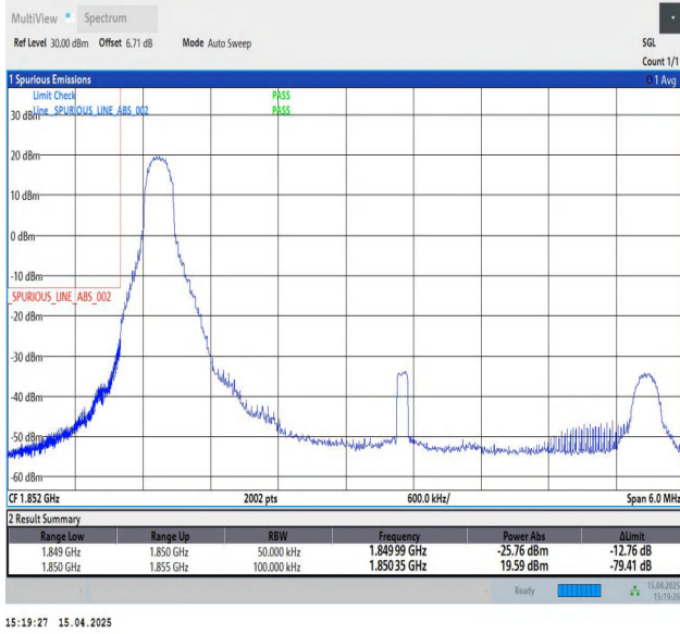
Band2-5MHz-QPSK-18625-1RB#0-PASS
