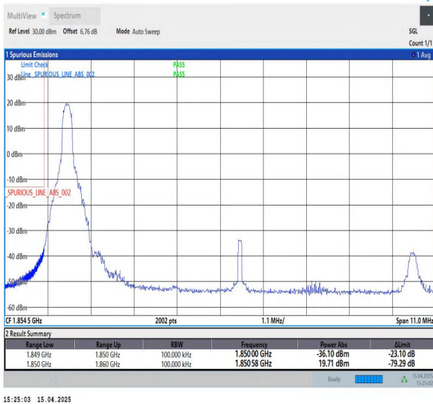
Band2-10MHz-QPSK-18650-1RB#0-PASS
