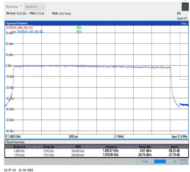
Band2-20MHz-QPSK-19100-100RB#0-PASS
