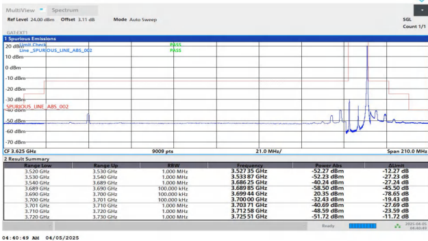
Band48-10MHz-QPSK-56690-1RB#49-PASS
