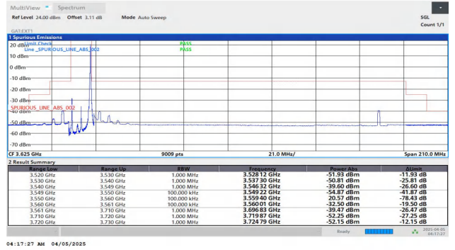
Band48-10MHz-QPSK-55290-1RB#49-PASS
