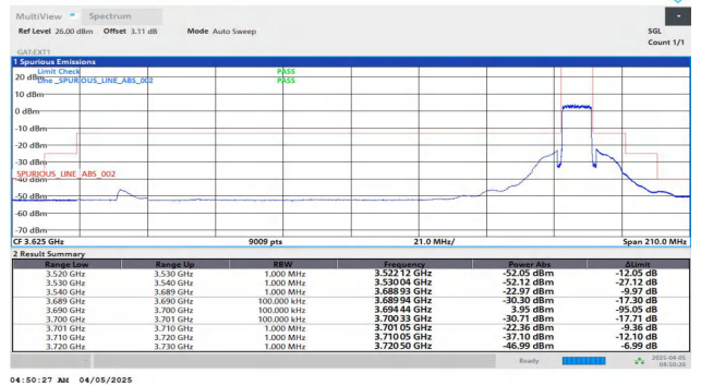
Band48-10MHz-QPSK-56690-50RB#0-PASS
