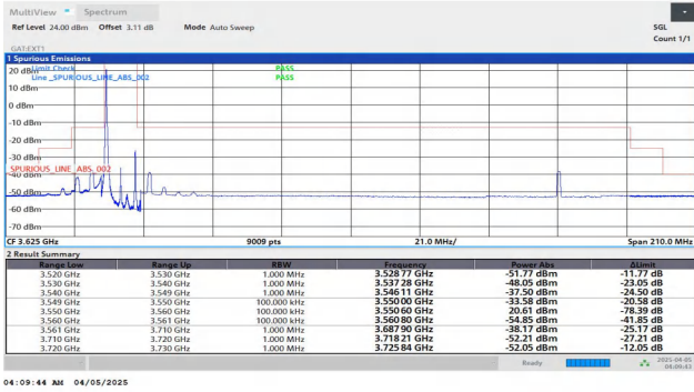
Band48-10MHz-QPSK-55290-1RB#0-PASS
