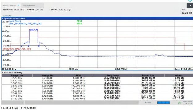
Band48-10MHz-QPSK-55290-50RB#0-PASS
