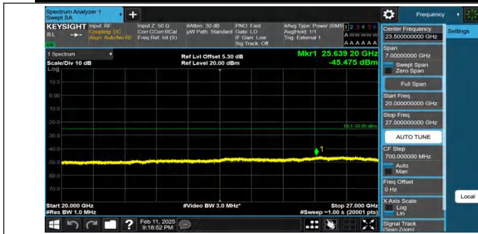
Band41-15MHz-QPSK-39725-1RB#0-20000~27000-PASS
