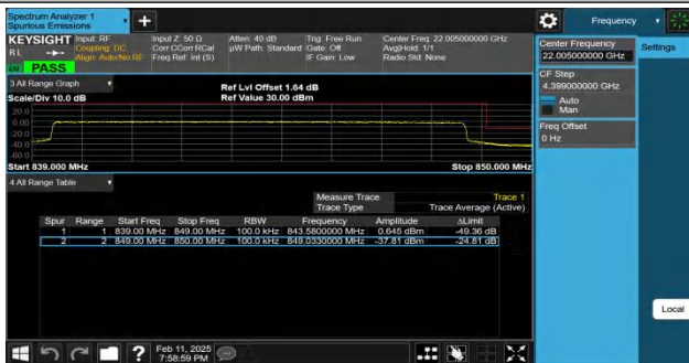
Band26(824-849)-10MHz-QPSK-26990-50RB#0-PASS
