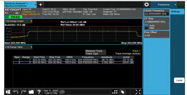
Band26(824-849)-10MHz-QPSK-26840-50RB#0-PASS
