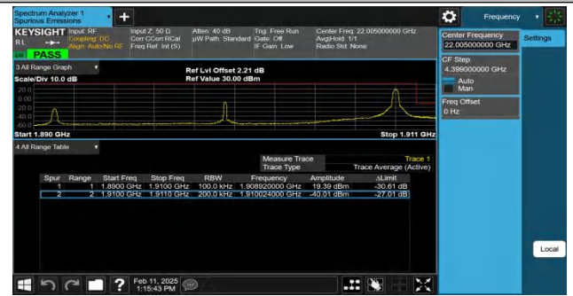
Band2-20MHz-QPSK-19100-1RB#99-PASS
