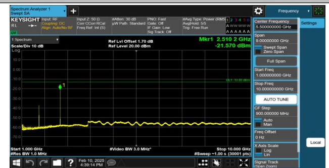
GPRS850-190-5-1000~10000MHz-PASS
