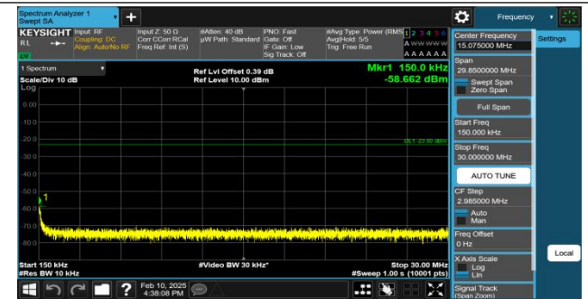
GPRS850-128-5-0.15~30MHz-PASS
