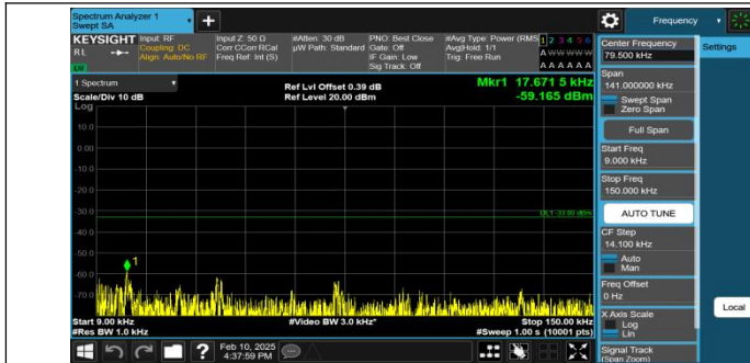
GPRS850-128-5-0.009~0.15MHz-PASS
