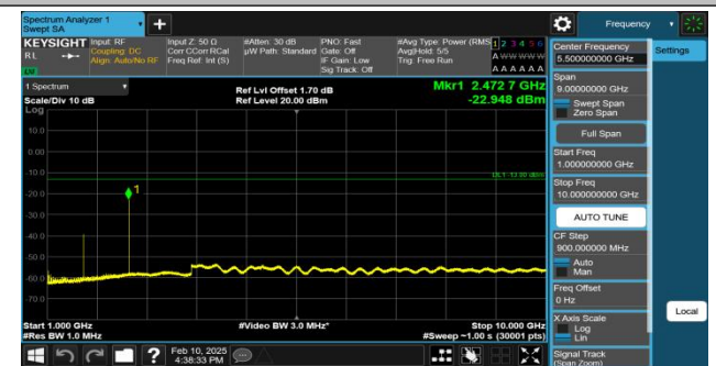
GPRS850-128-5-1000~10000MHz-PASS
