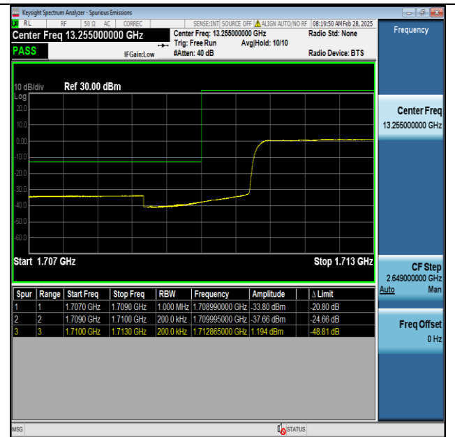
Band4-20MHz-QPSK-20050-100RB#0-PASS
