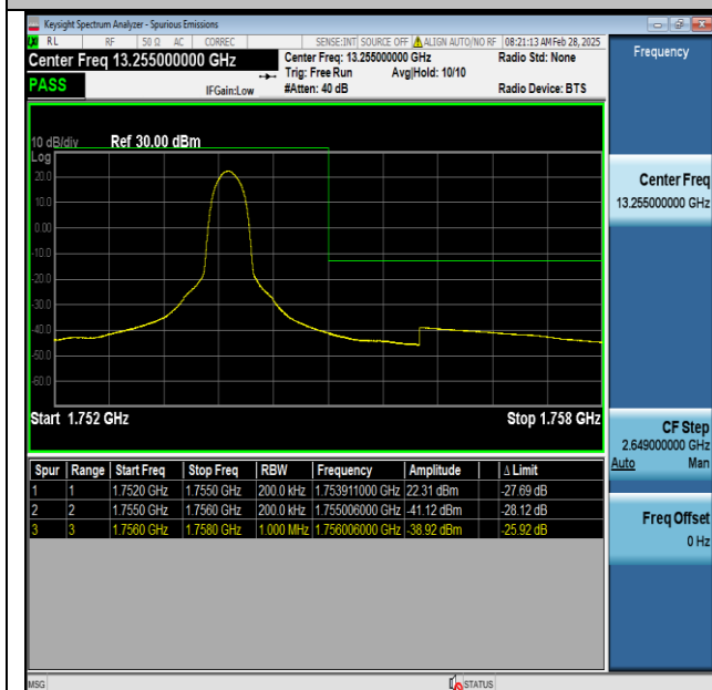
Band4-20MHz-QPSK-20300-1RB#99-PASS
