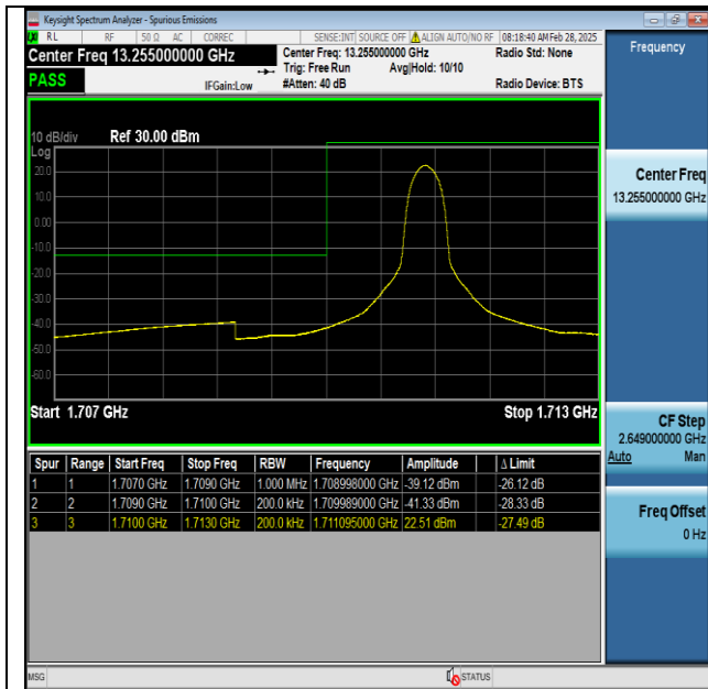
Band4-20MHz-QPSK-20050-1RB#0-PASS
