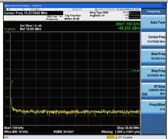
Band II-9538-0.15~30MHz-PASS
