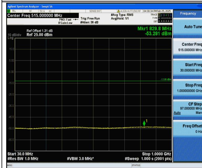
Band II-9538-30~1000MHz-PASS
