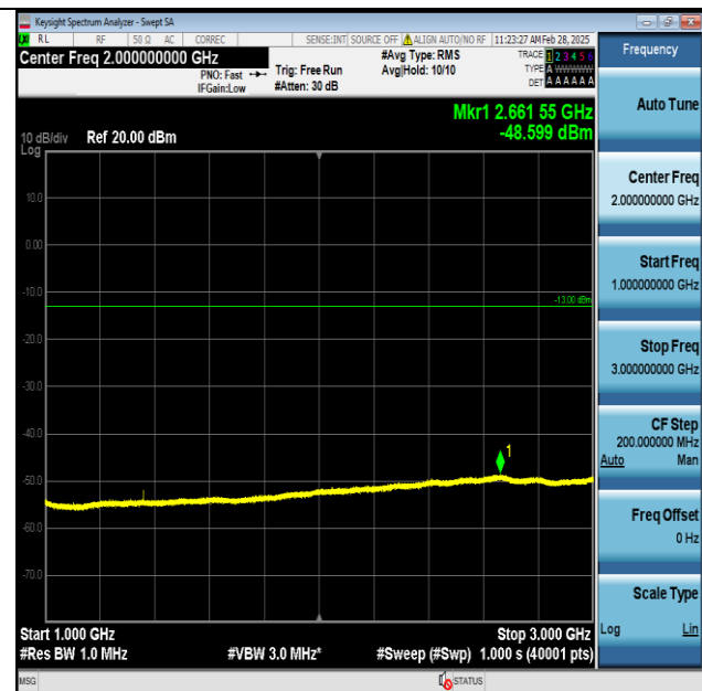
Band71-20MHz-QPSK-133372-1RB#0-1000~3000-PASS
