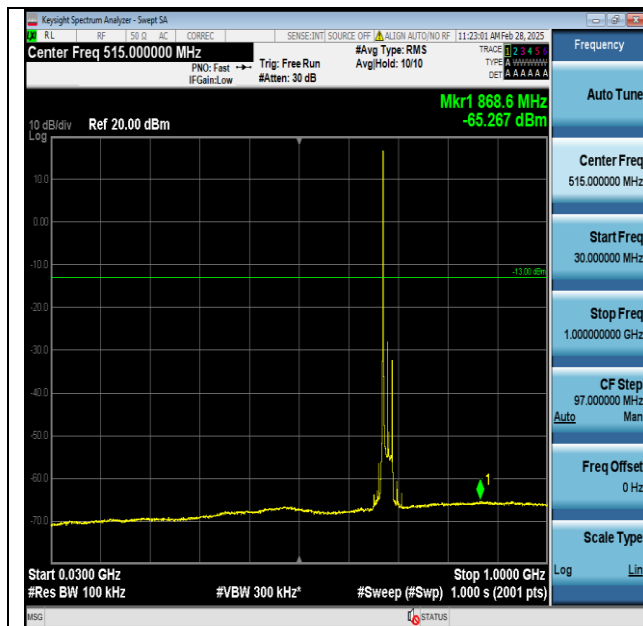
Band71-20MHz-QPSK-133372-1RB#0-30~1000-PASS
