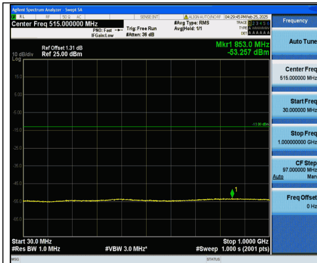
Band II-9400-30~1000MHz-PASS
