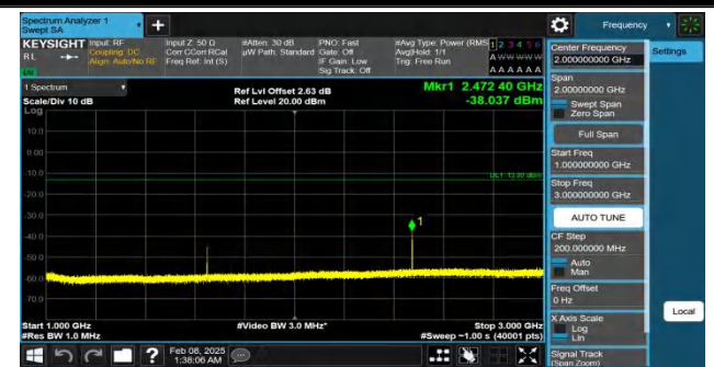
Band26(824-849)-3MHz-QPSK-26805-1RB#0-1000~3000-PASS
