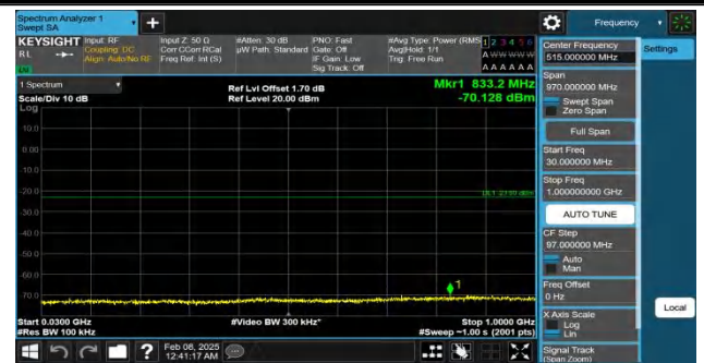
Band25-20MHz-QPSK-26590-1RB#99-30~1000-PASS
