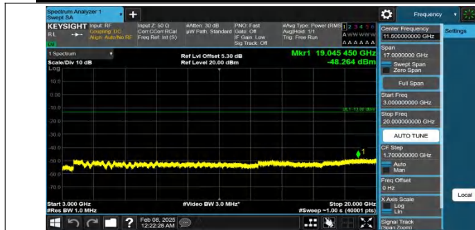
Band25-10MHz-QPSK-26365-1RB#0-3000~20000-PASS
