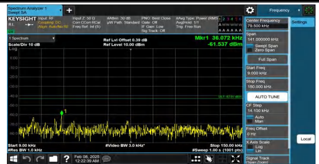
Band25-10MHz-QPSK-26365-1RB#49-0.009~0.15-PASS
