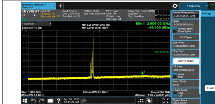
Band25-20MHz-QPSK-26590-1RB#99-1000~3000-PASS
