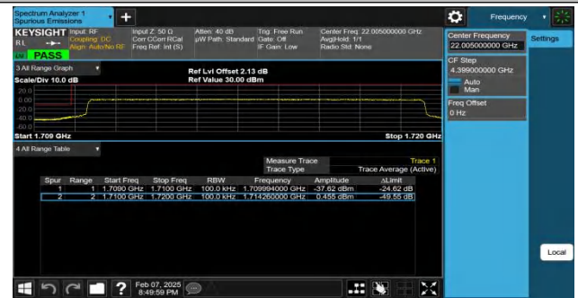
Band4-10MHz-QPSK-20000-50RB#0-PASS
