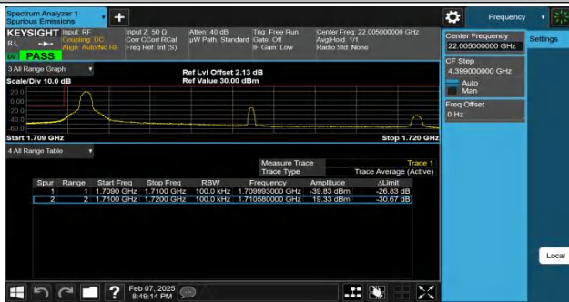
Band4-10MHz-QPSK-20000-1RB#0-PASS
