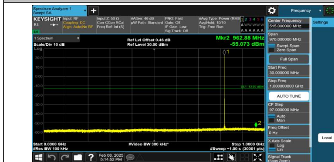
GPRS850-128-5-30~1000MHz-PASS
