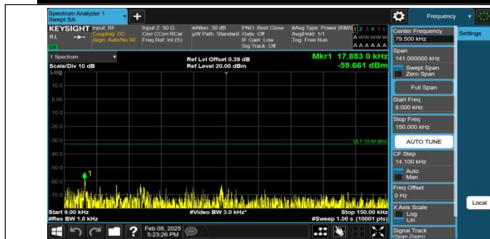
EGPRS850-190-8-0.009~0.15MHz-PASS
