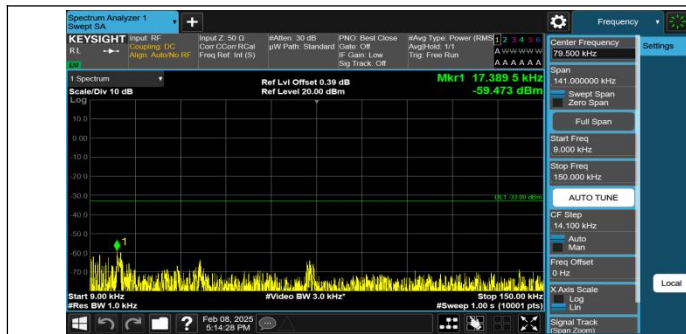
GPRS850-128-5-0.009~0.15MHz-PASS
