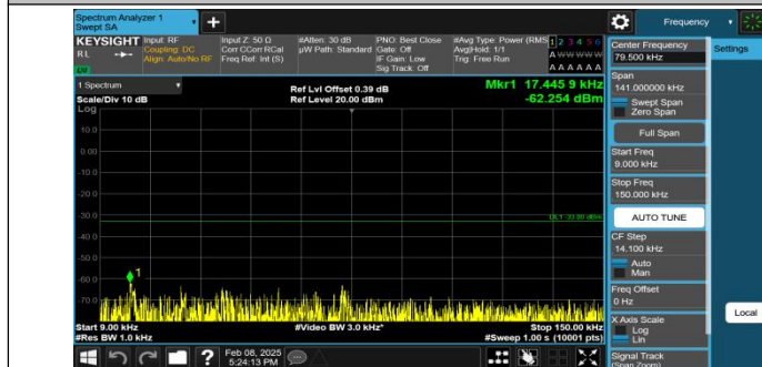
EGPRS850-251-8-0.009~0.15MHz-PASS
