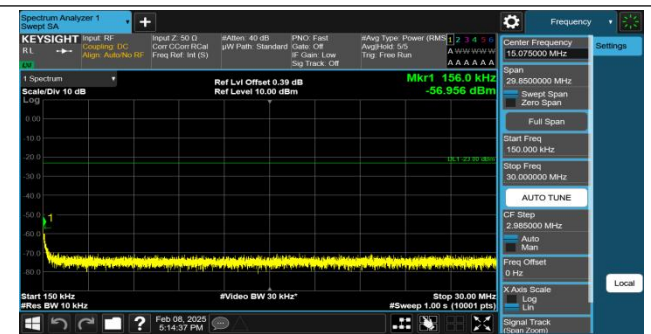
GPRS850-128-5-0.15~30MHz-PASS
