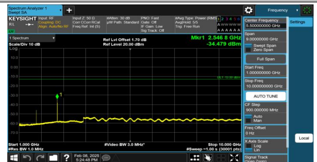
EGPRS850-251-8-1000~10000MHz-PASS
