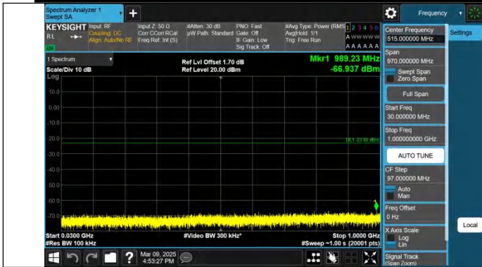
Band2-20MHz-QPSK-18700-1RB#0-30~1000-PASS
