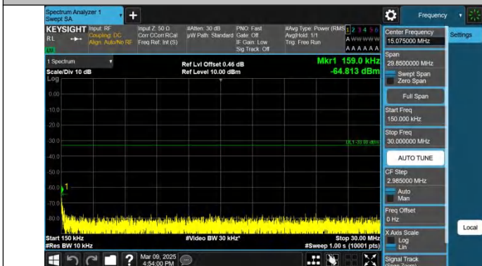
Band2-20MHz-QPSK-18700-1RB#99.0.15~30-PASS
