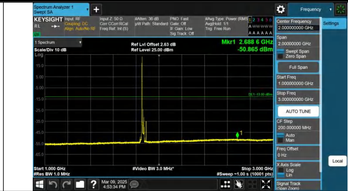
Band2-20MHz-QPSK-18700-1RB#0-1000~3000-PASS
