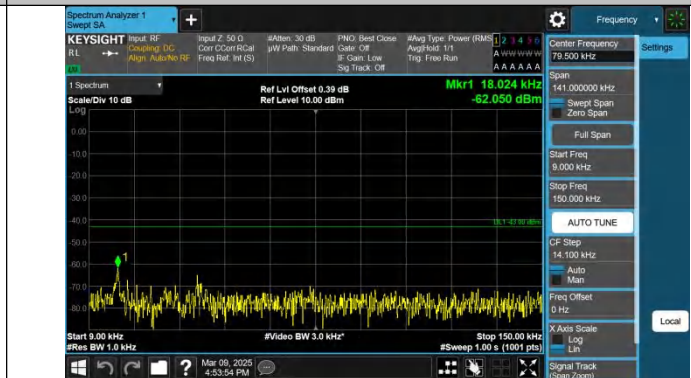
Band2-20MHz-QPSK-18700-1RB#99.0.009~0.15-PASS
