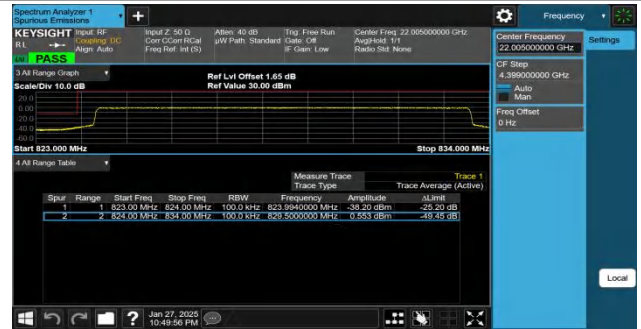
Band26(824-849)-10MHz-QPSK-26840-50RB#0-PASS
