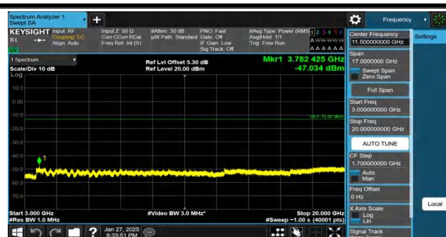
Band25-20MHz-QPSK-26365-1RB#99-3000~20000-PASS
