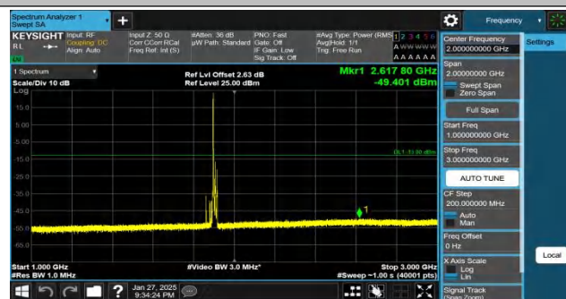
Band25-20MHz-QPSK-26590-1RB#0-1000~3000-PASS
