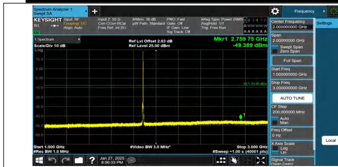
Band25-3MHz-QPSK-26365-1RB#14-1000~3000-PASS
