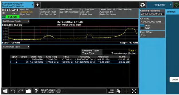
Band4-3MHz-QPSK-19965-1RB#14-PASS
