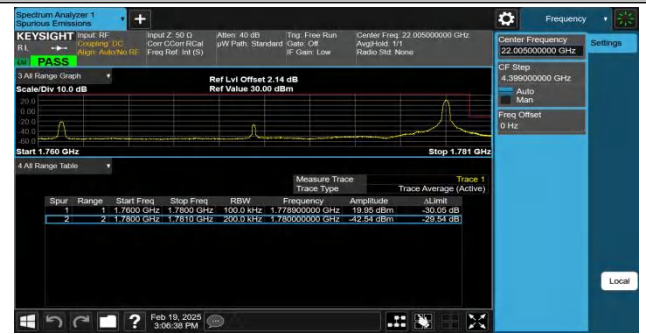
Band66-20MHz-QPSK-132572-1RB#99-PASS
